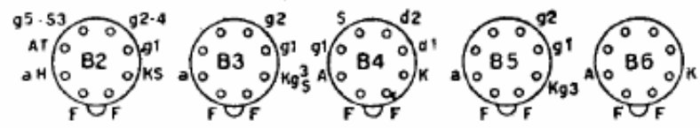
PHILIPS RADIO - Mod. BI 210 A. Onde corte a 16,5 Mc e 8 Mc. Onde medie a 550 kc e 1630 kc/s. Media frequenza 468 kc. Corrente totale 68 mA. Consumo totale 32 watt.
