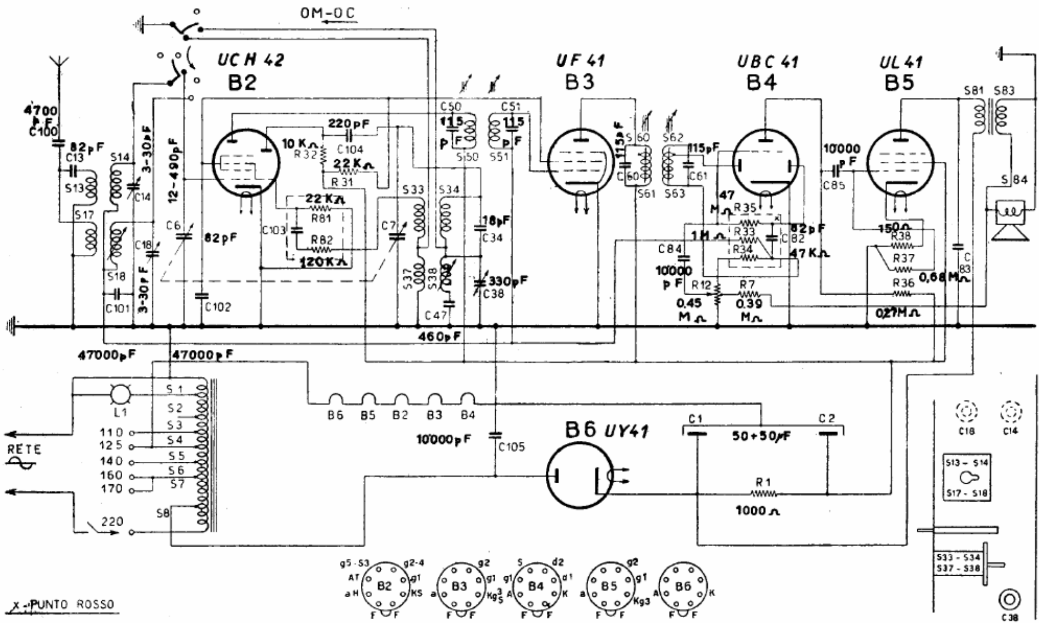
PHILIPS RADIO - Mod. BI 210 A. Onde corte a 16,5 Mc e 8 Mc. Onde medie a 550 kc e 1630 kc/s. Media frequenza 468 kc. Corrente totale 68 mA. Consumo totale 32 watt.
